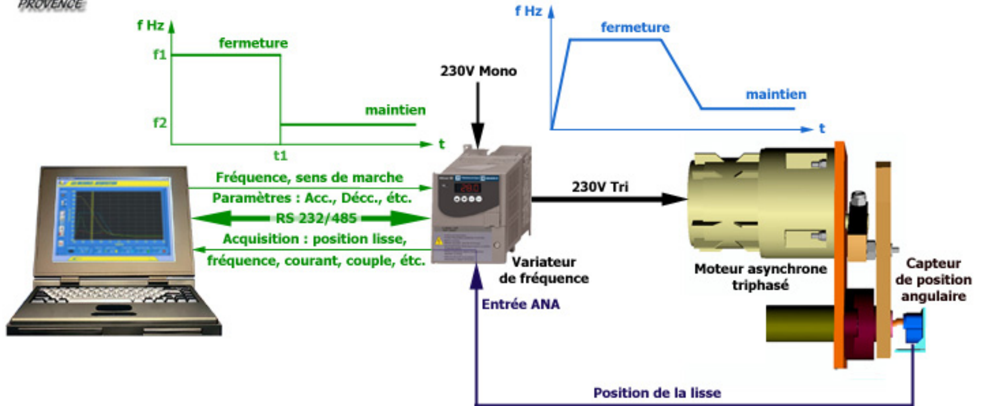
Synoptique partie commande barrière SYMPACT version didactisée
