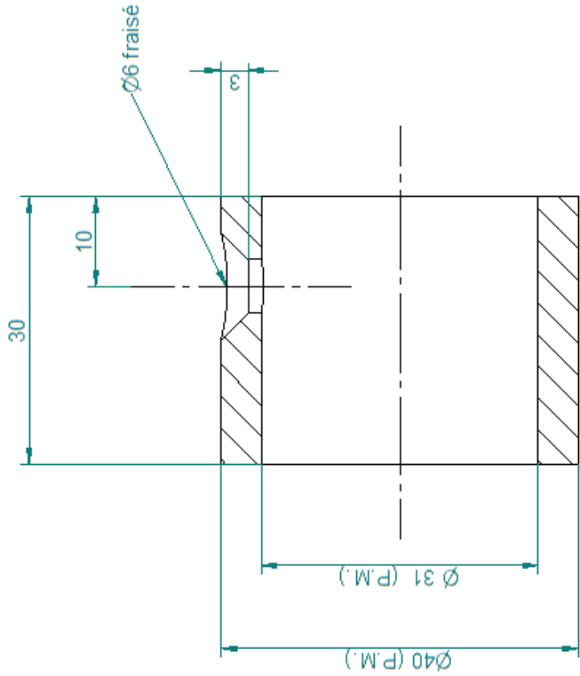
Coupe A-A
