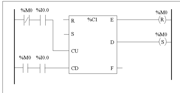
Schéma à contacts
