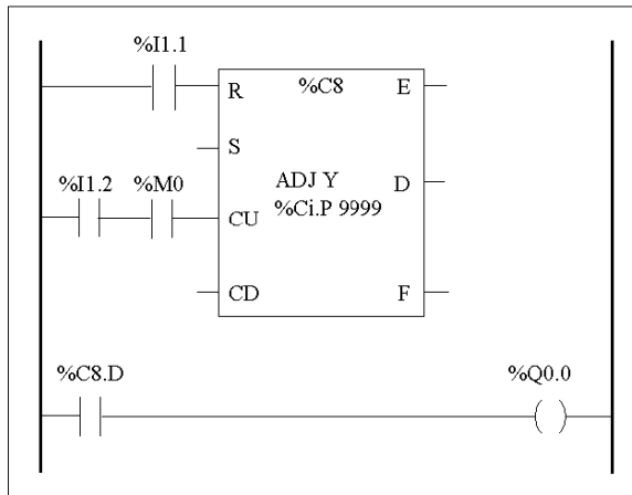
Schéma à contacts
