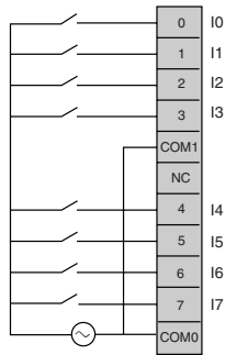
Câblage d'entrée 120 VAC
