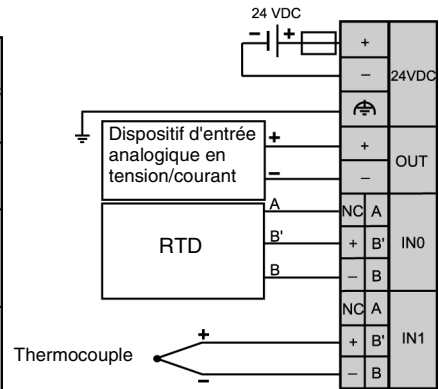
Câblage 3 fils :
