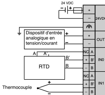
Câblage 4 fils :
