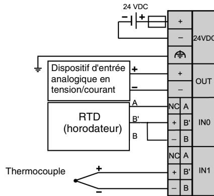
Câblage 2 fils :
