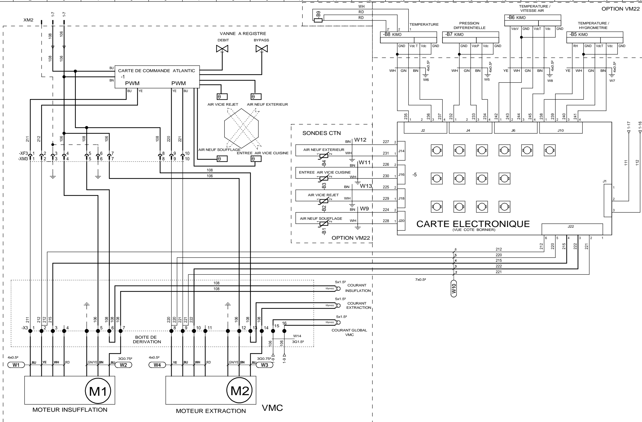
VM20-VMC DOUBLE FLUX INSTRUMENTÉE SCHEMA ELECTRIQUE
