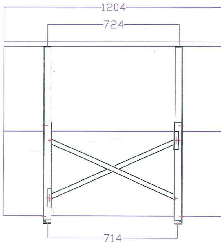
VUE ARRIERE
