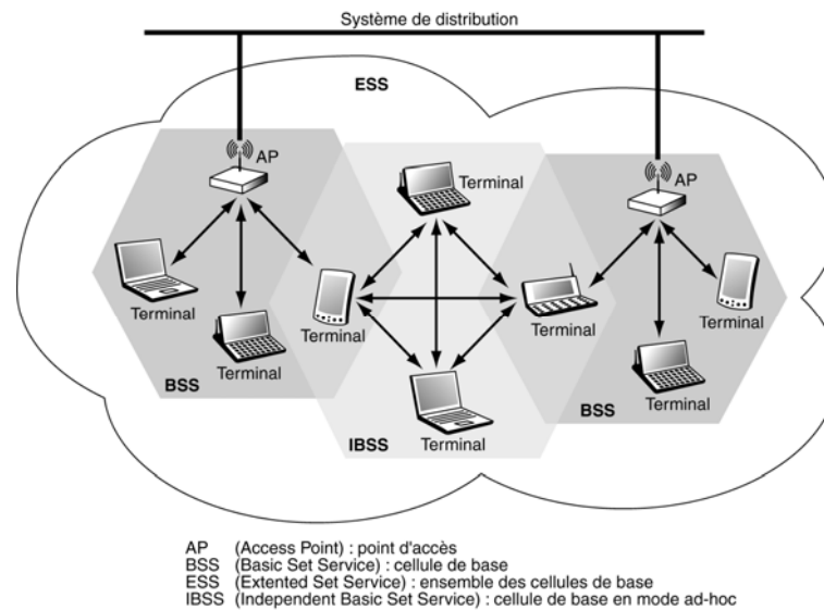
Figure 62. Architecture d'un réseau Wi-Fi.
