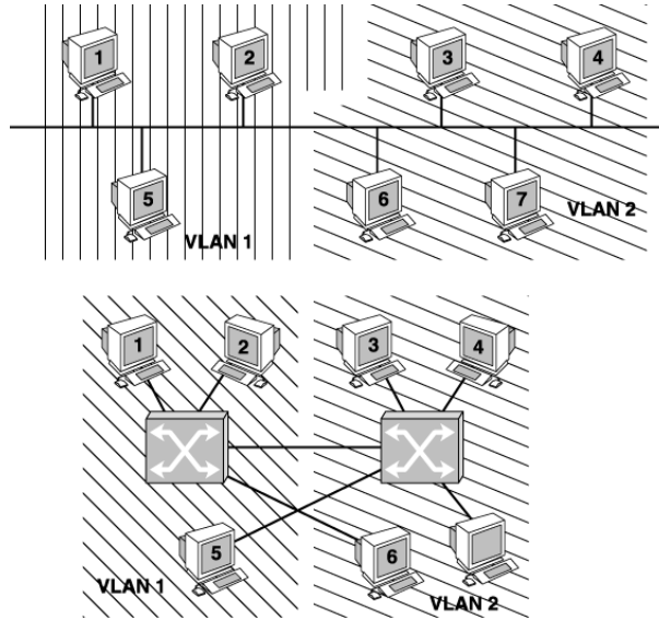
Figure 36. Deux topologies de VLAN
