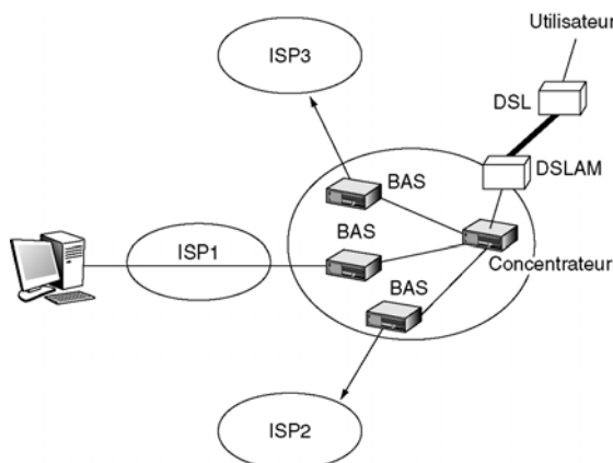
Figure 68 Équipements de concentration entre l'utilisateur et le serveur
